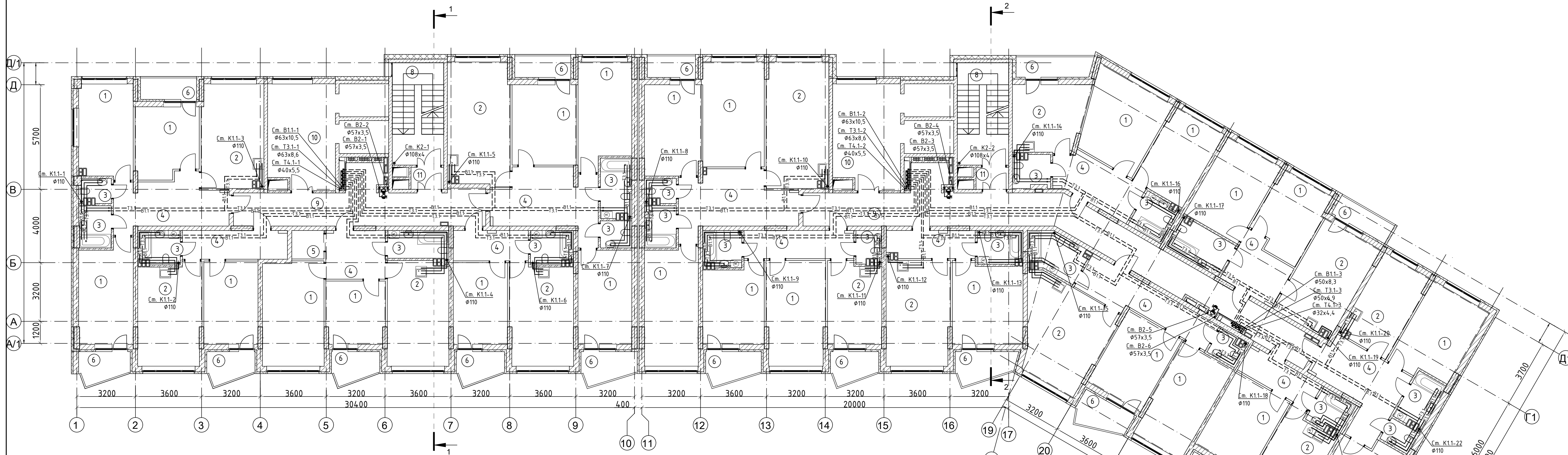
Экспликация помещений 5-10 этажей
