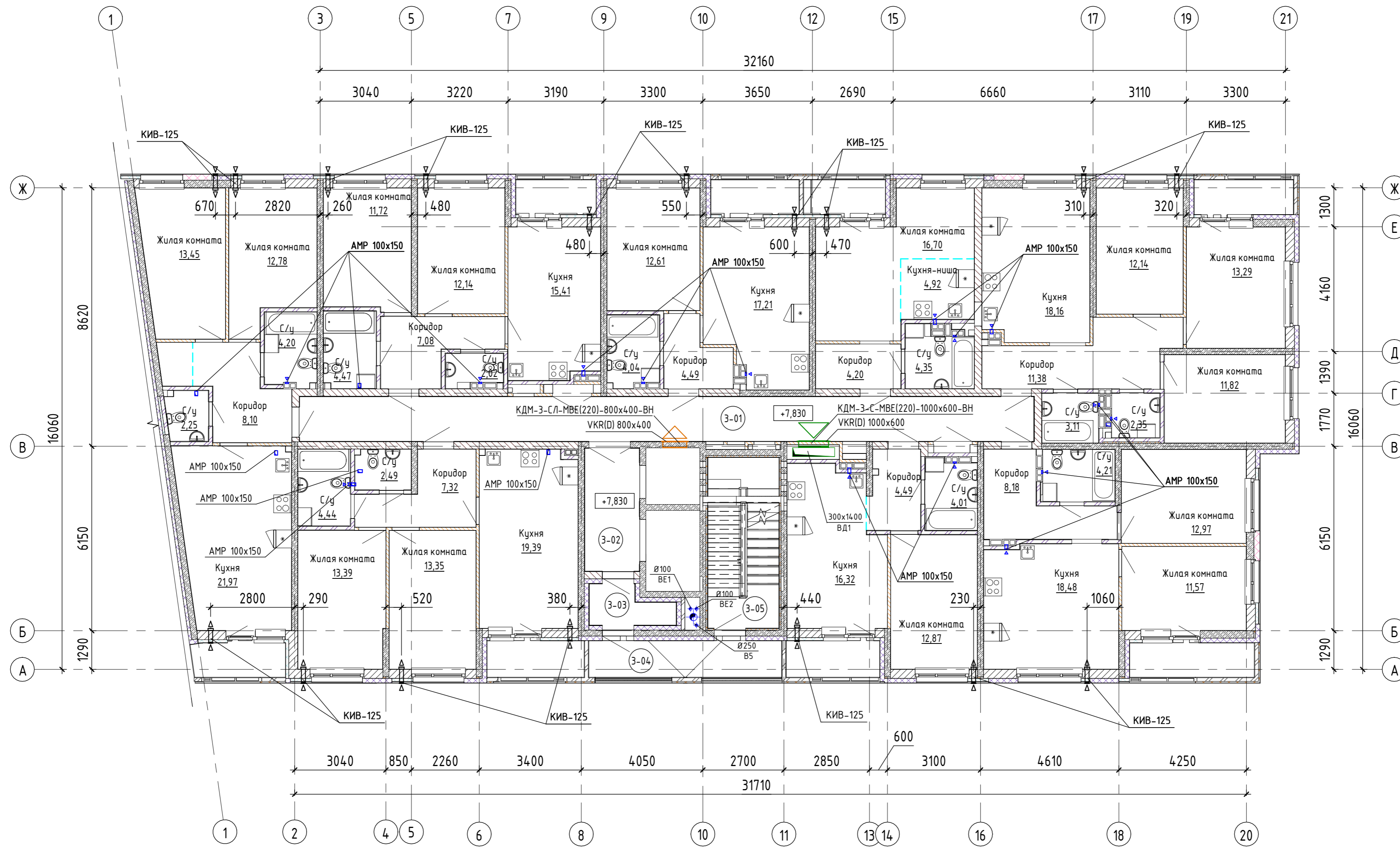
Экспликация помещений
