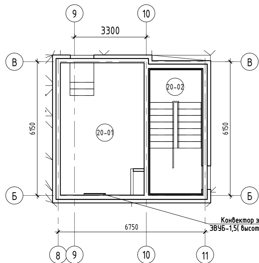
План машинного помещения
